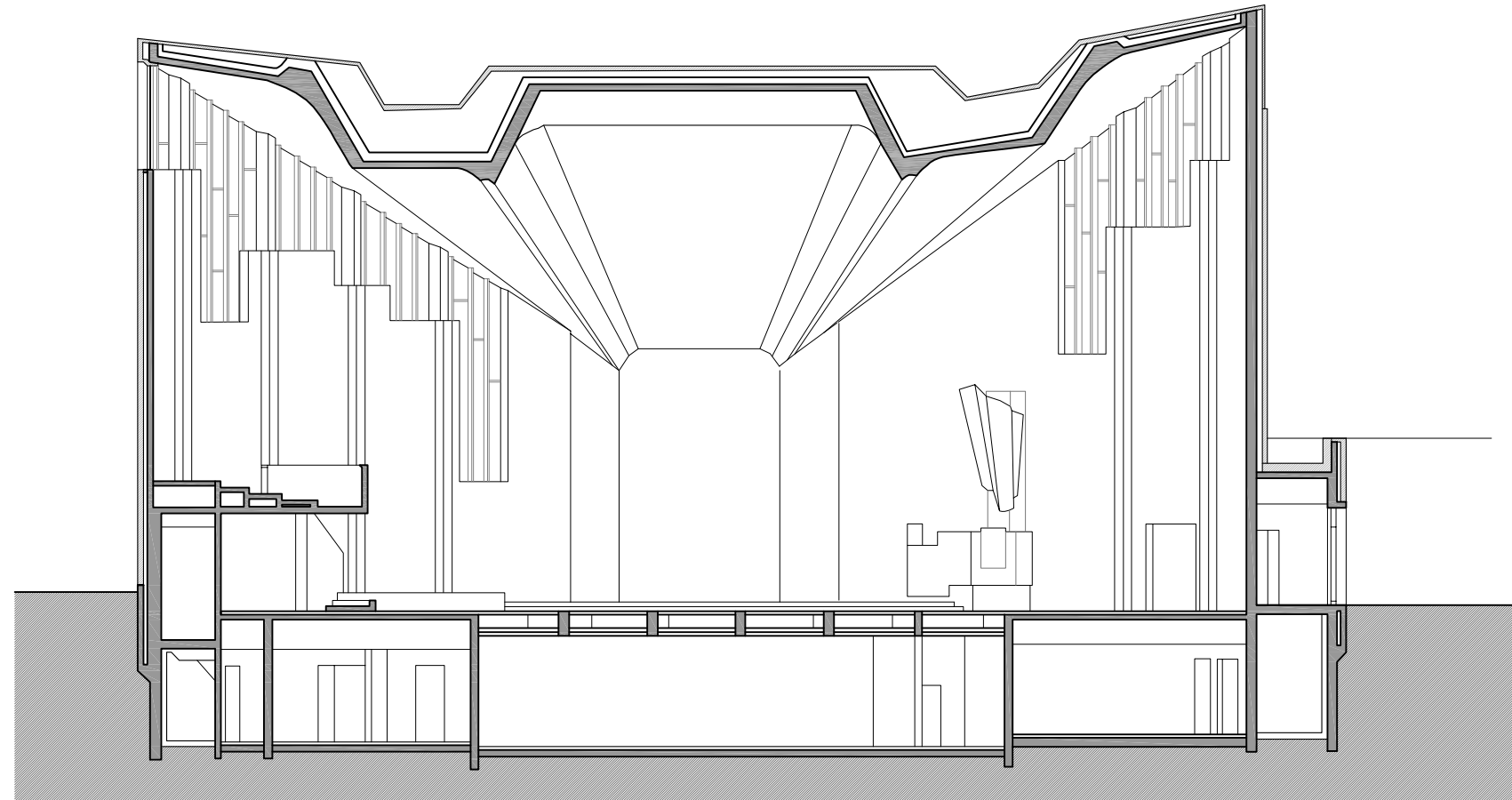
Secció B-B'
