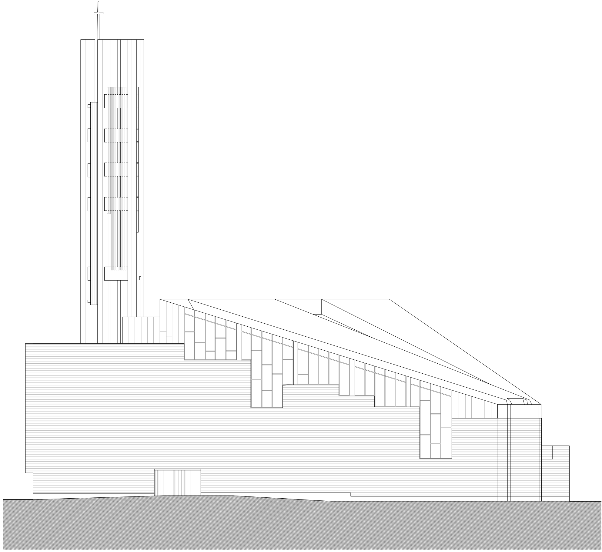
Alçat Est
