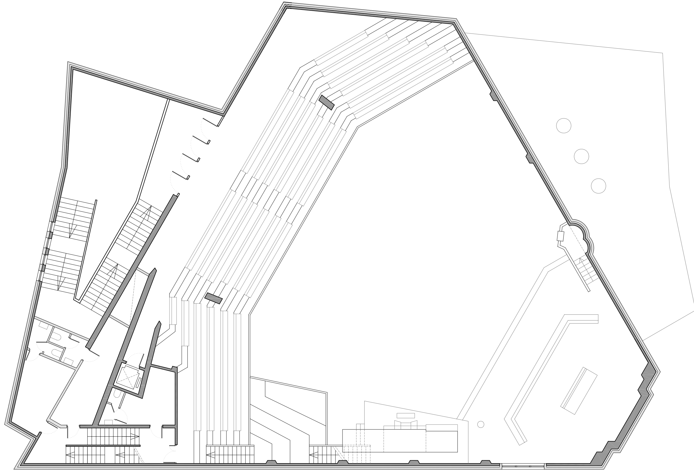
Planta Primera
