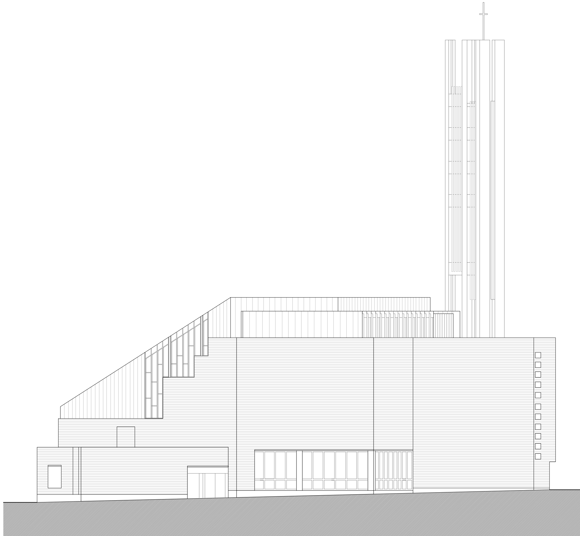
Alçat Oest
