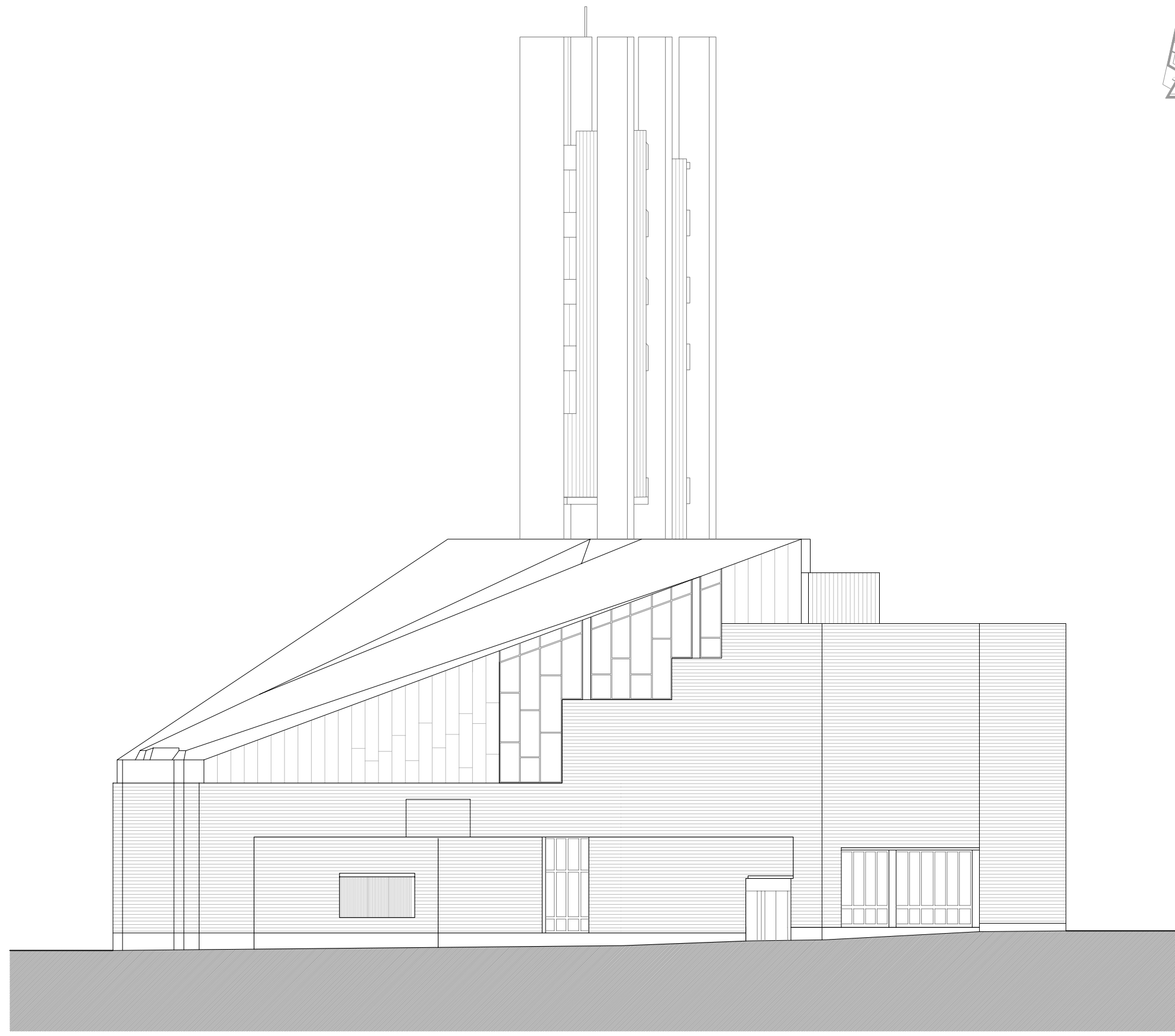
Alçat Nord
