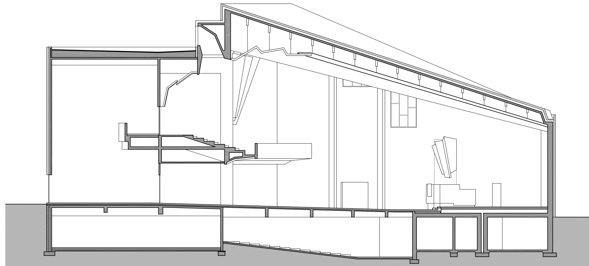
Secció A-A'
