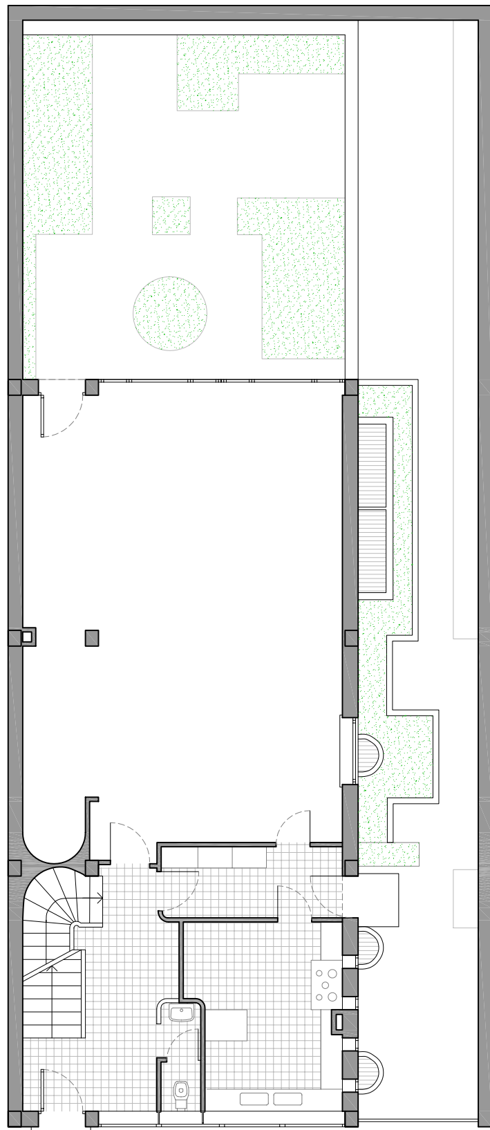
Planta baixa
