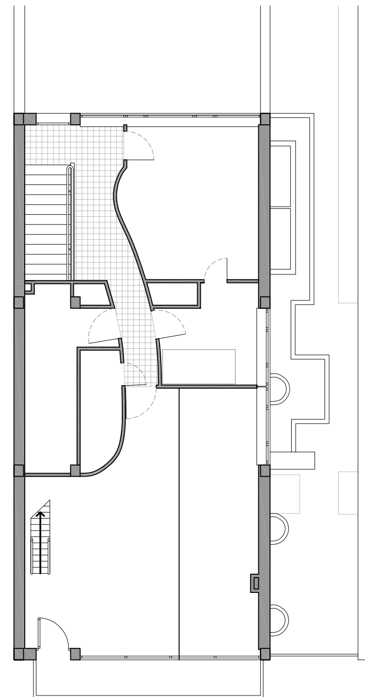
Planta segona
