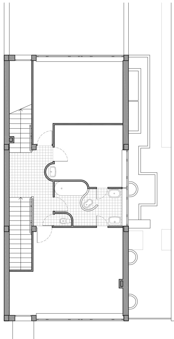
Planta primera
