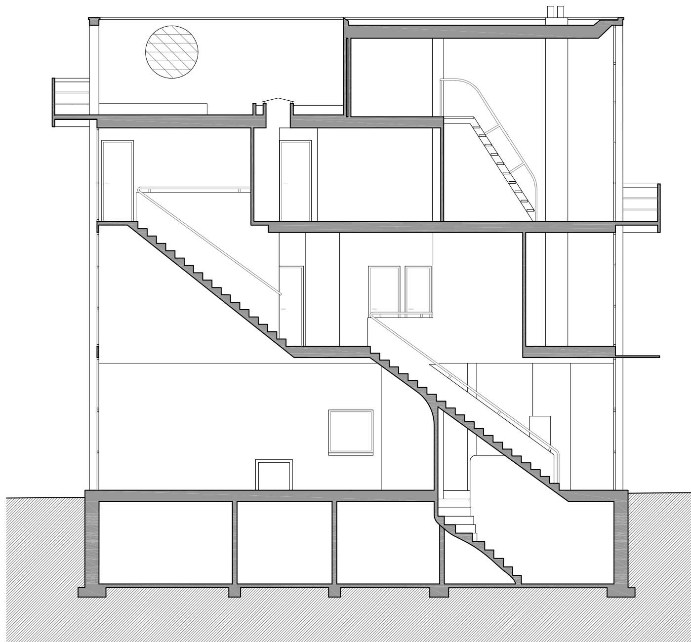
Secció a-a'
