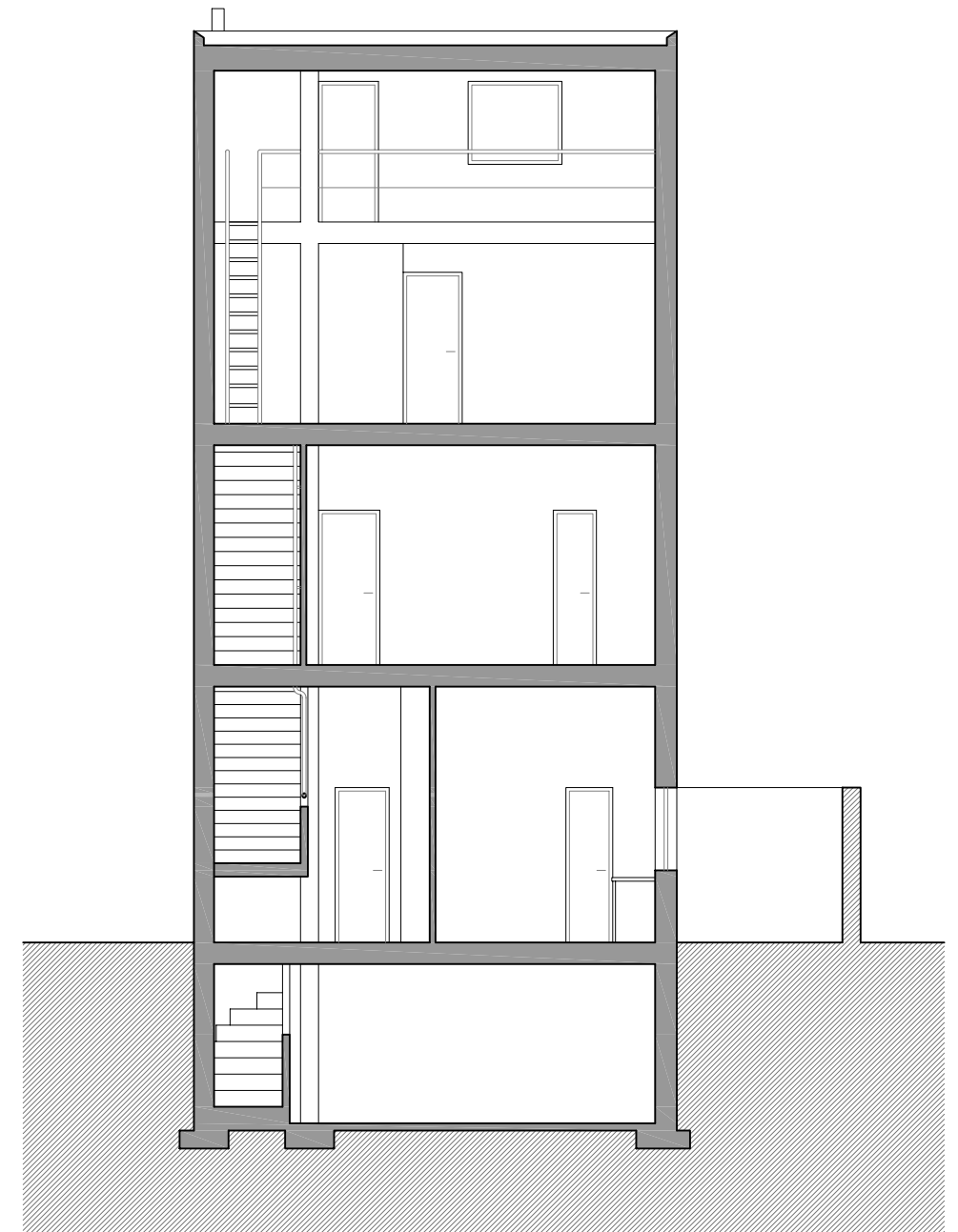
Secció transversal
