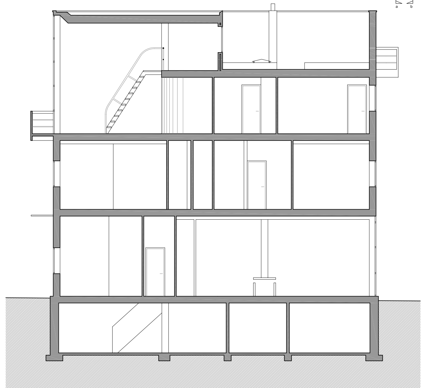
Secció b-b'
