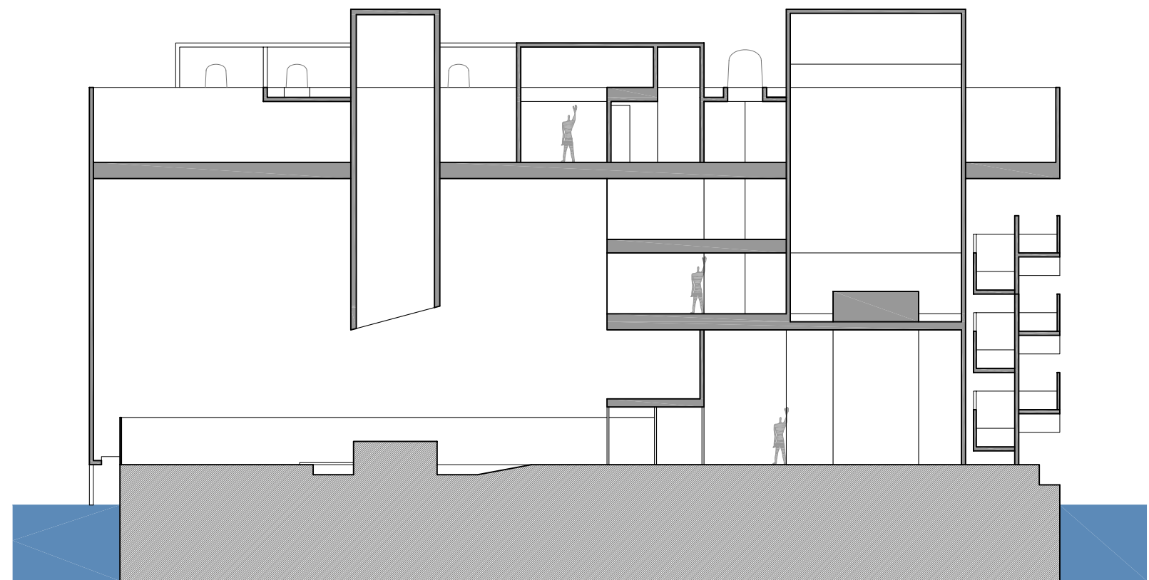
Secció longitudinal
