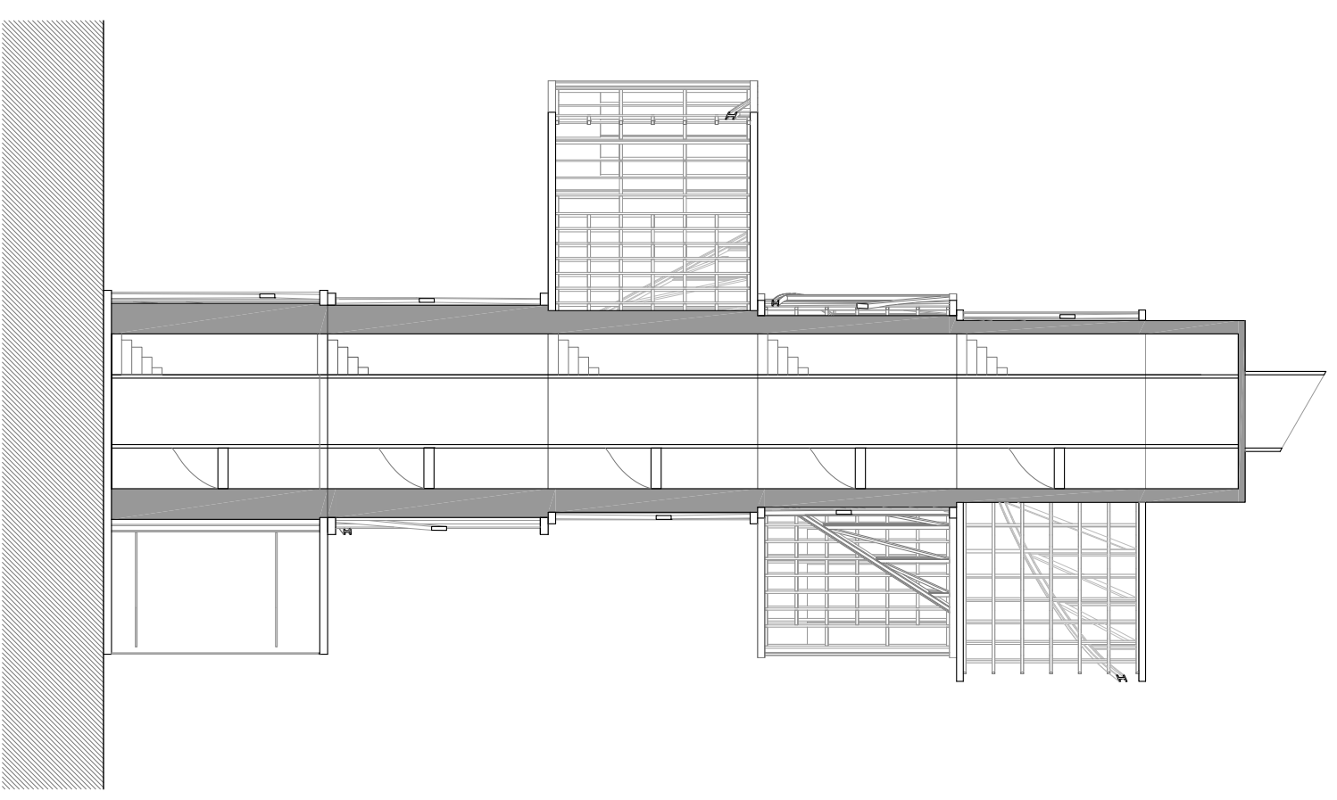
Secció
